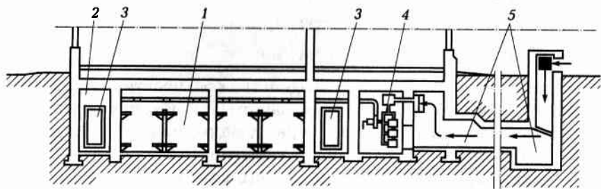
Рис. 1.2. Противорадиационное укрытие: 1 — отсеки для укрываемых людей; 2 — тамбур; 3 — защитно-герметические двери; 4 — фильтровентиляционная установка; 5 — аварийный выход, используемый для забора воздуха
